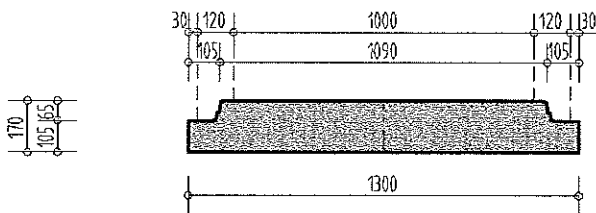
Betonschachtbodenplatte Dn 1000/170mm GRD
