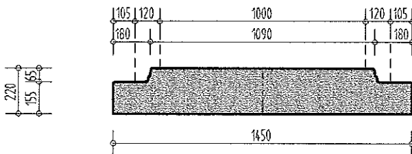
Betonschachtbodenplatte Dn 1000/220mm GRD
