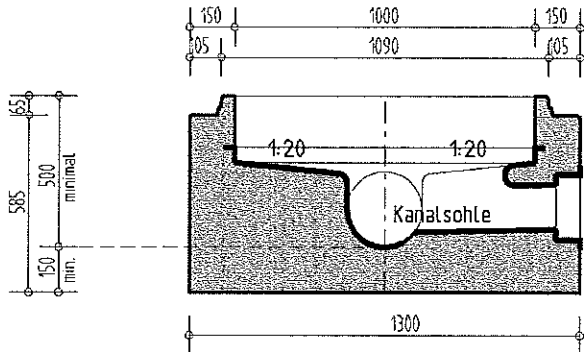
Betonschachtboden Dn 1000mm GRD
